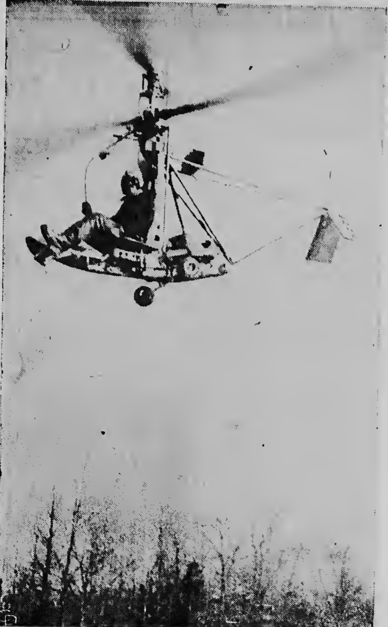
Het laatste nieuwtje op het gebied van helicopters: een 500-pond wegende, apklapbare wentelwiek. De Amerikaanse marine heeft er zesduizend besteld, ook voor landbouwers en andere particuliere instellingen zal de machine verkrijgbaar zijn.
